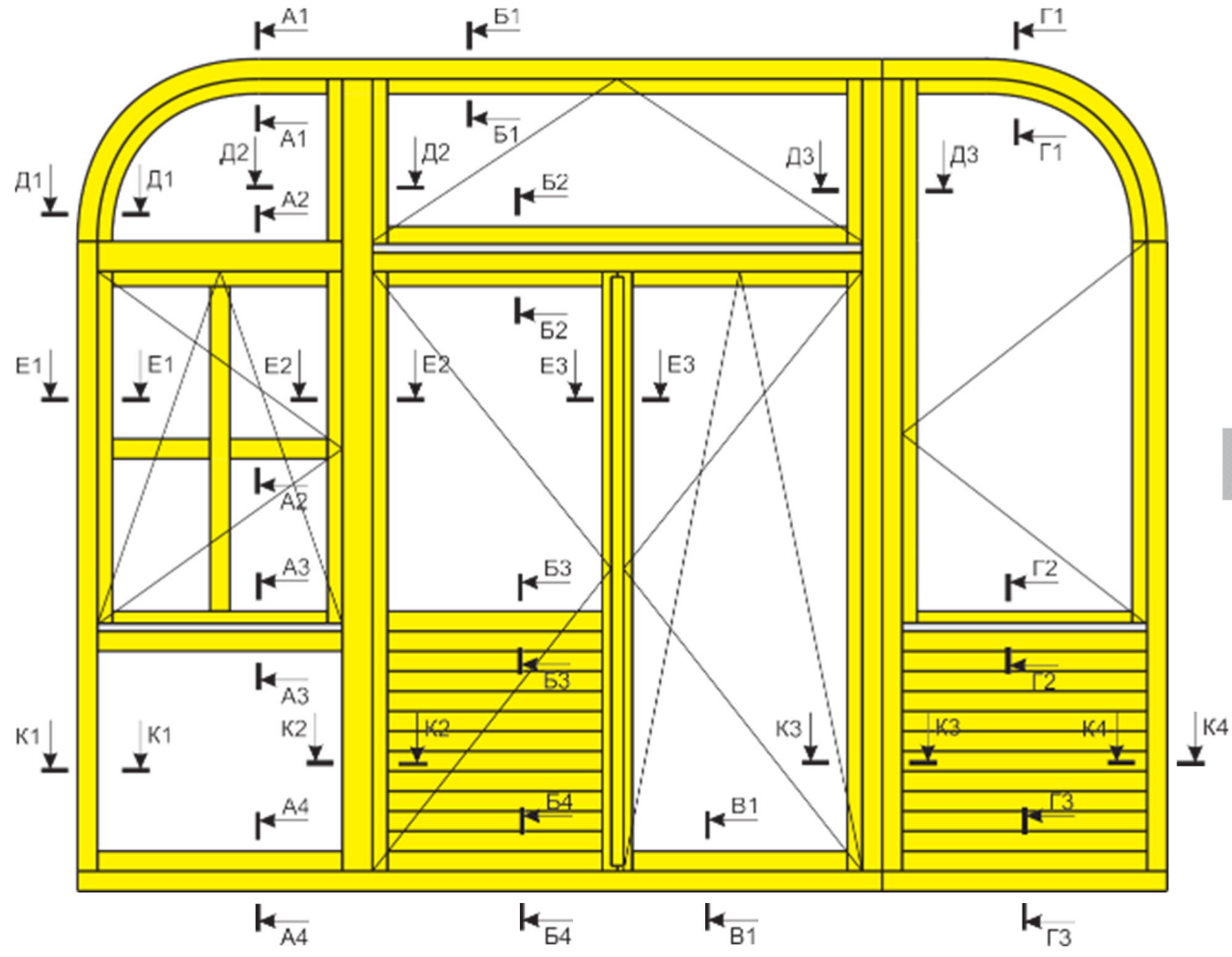
Горизонтальные разрезы
