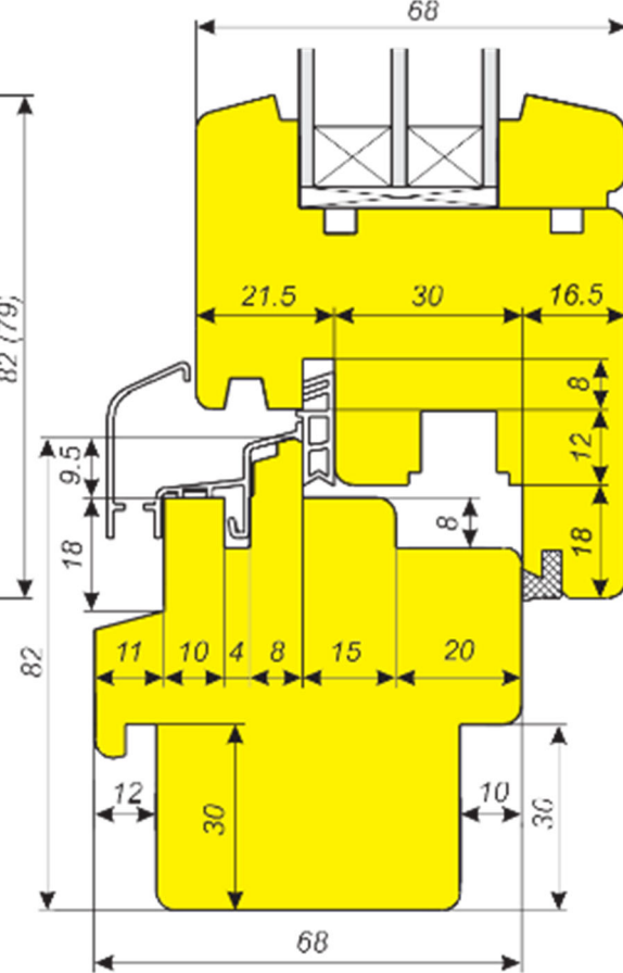
Вертикальное сечение окна из бруса на 68 мм
