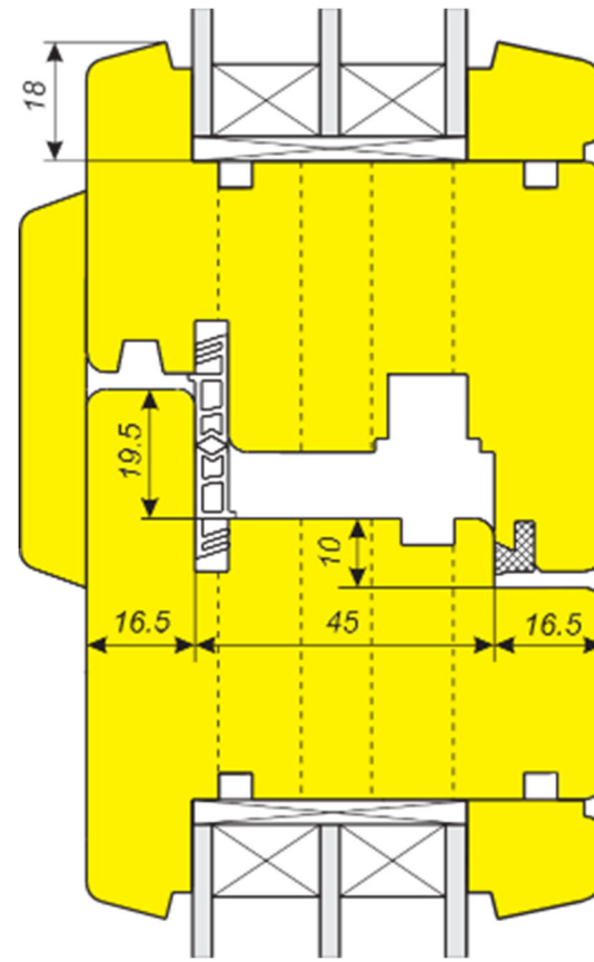
Сечение безимпостного притвора
