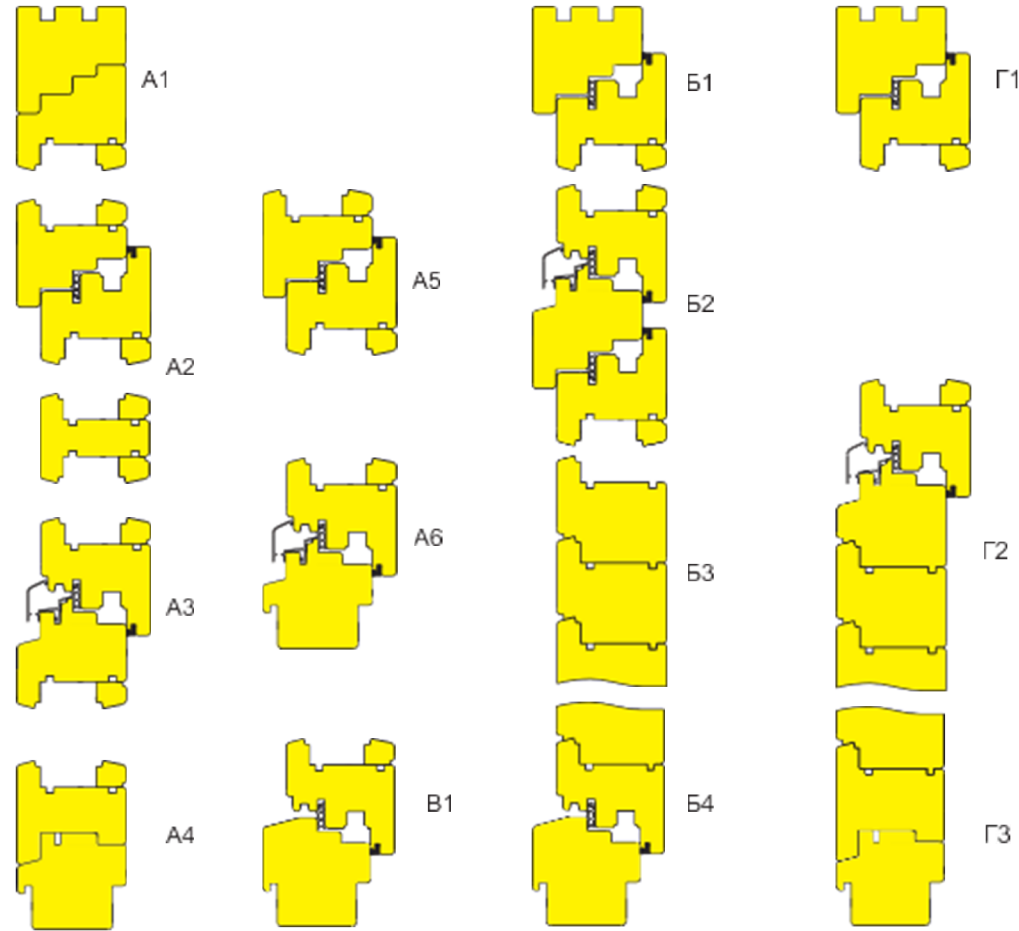
Вертикальные разрезы
