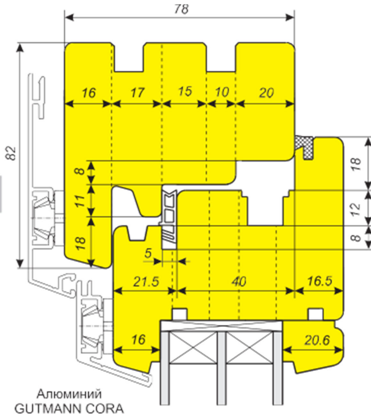
Вертикальное сечение
