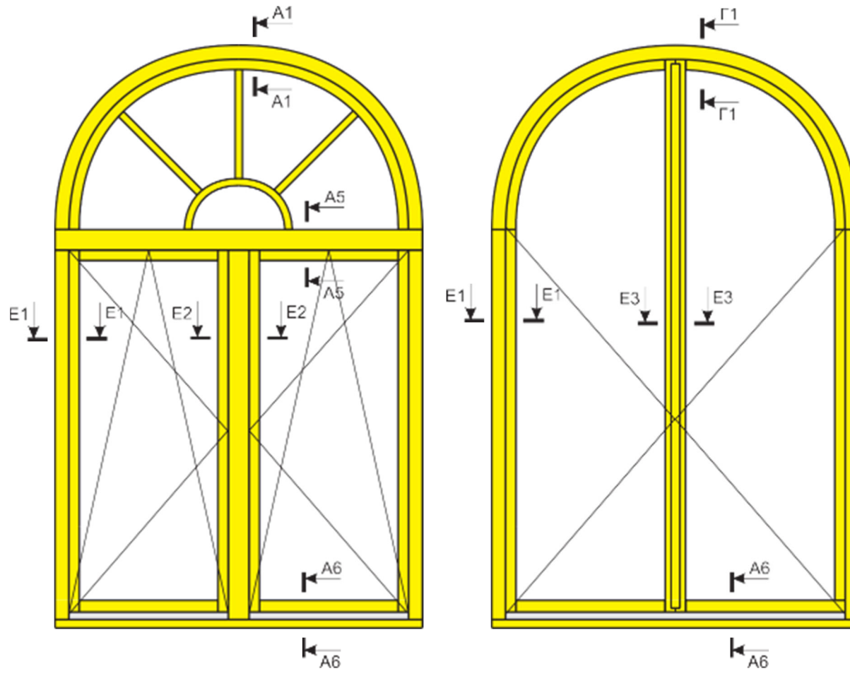
Вертикальные разрезы
